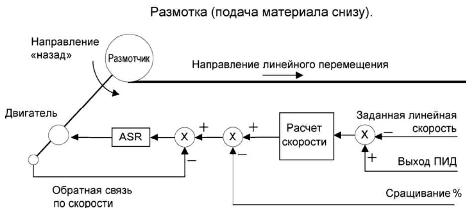
Рис 4. Размотка рулона при подаче материала снизу.
