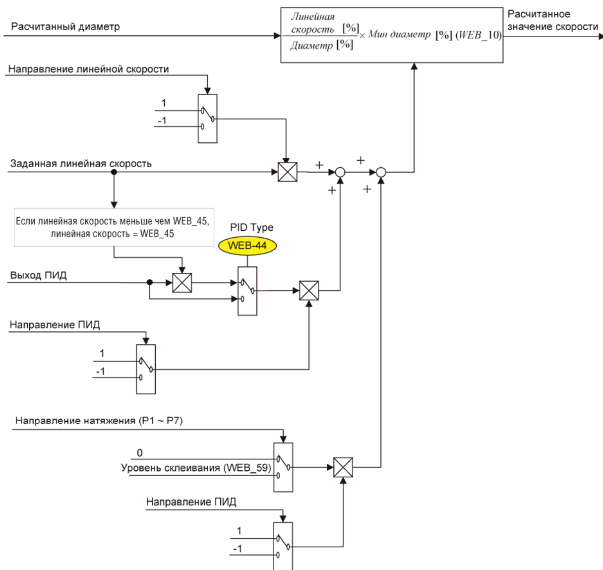
Функциональная схема расчета линейной скорости
