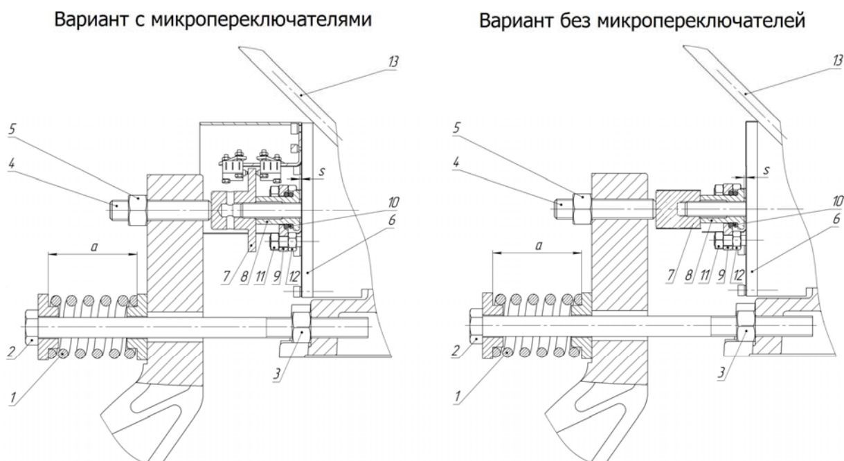
Рис. 21. Регулировка тормоза
