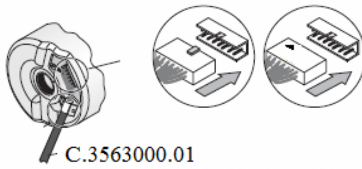
Рис. 7. Вид разъема датчика.
