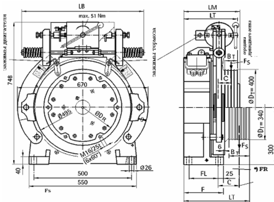
Рис. 2. Габаритные размеры.
