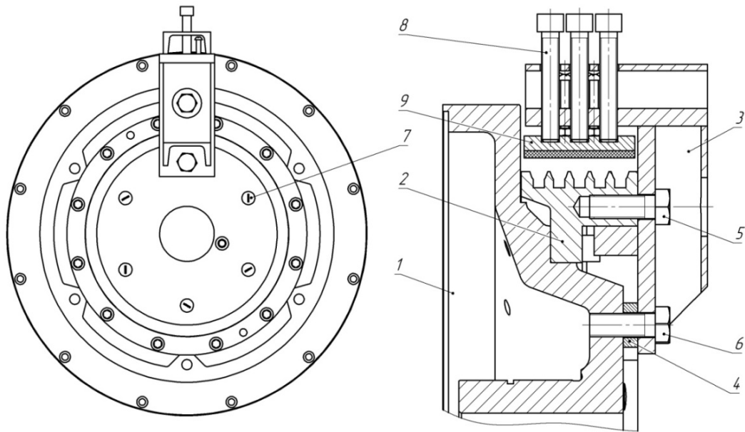
Рис. 15. Струбцина для лифтов БМП
