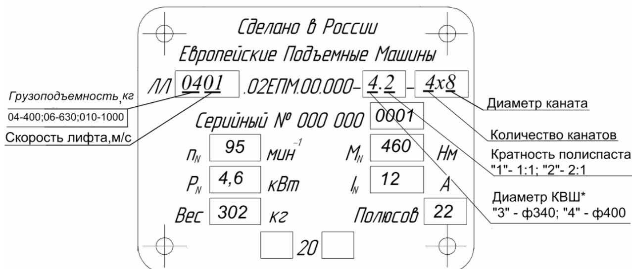
Рис. 1. Шильдик и маркировка лебедки.
