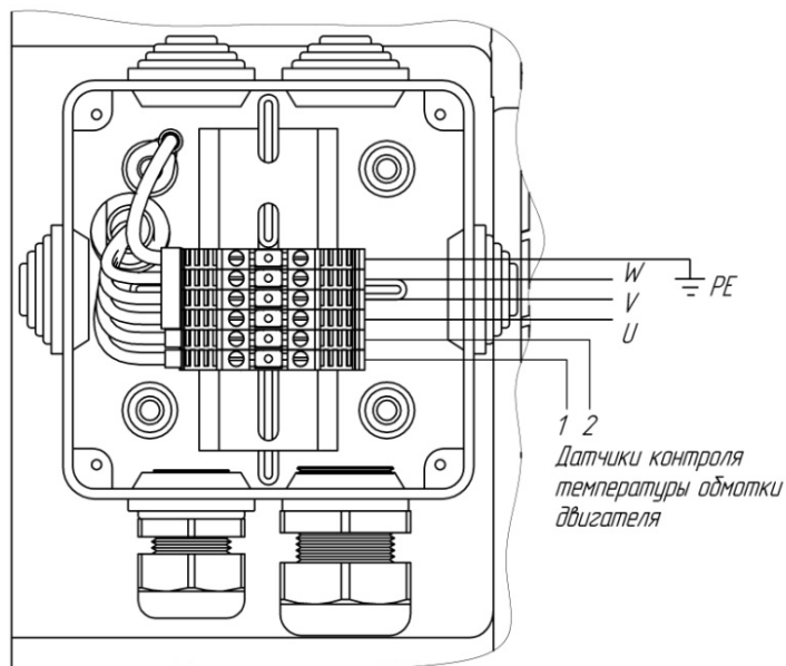
Рис. 19. Подключение двигателя
