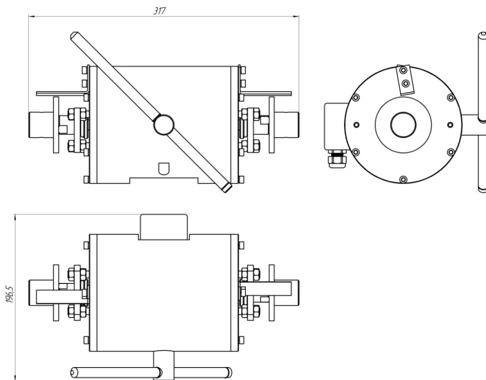
Рис. 4. Электромагнит выталкивающий
