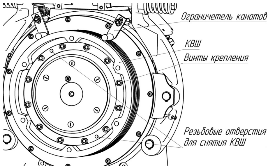
Рис. 26. Замена КВШ.
