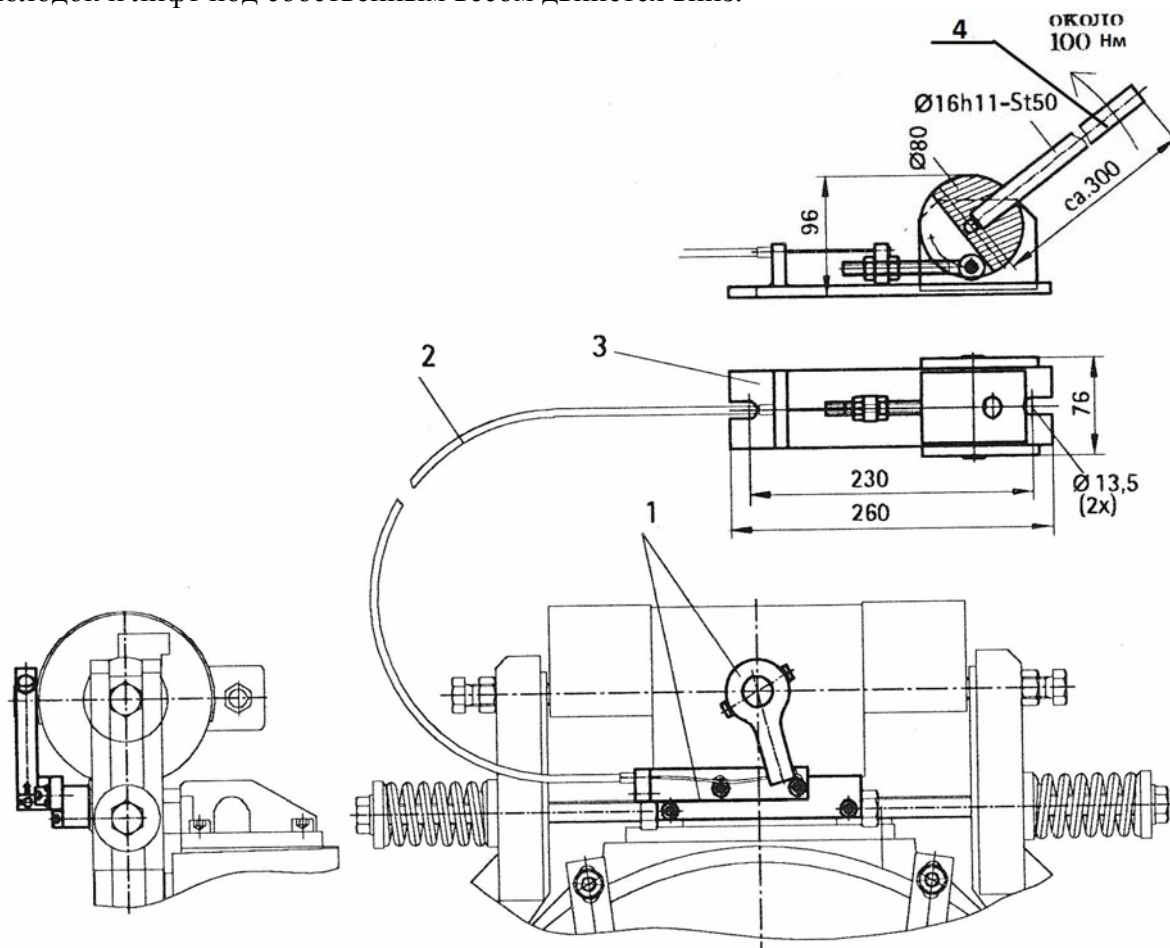
Рис. 14. Трос Бодена
