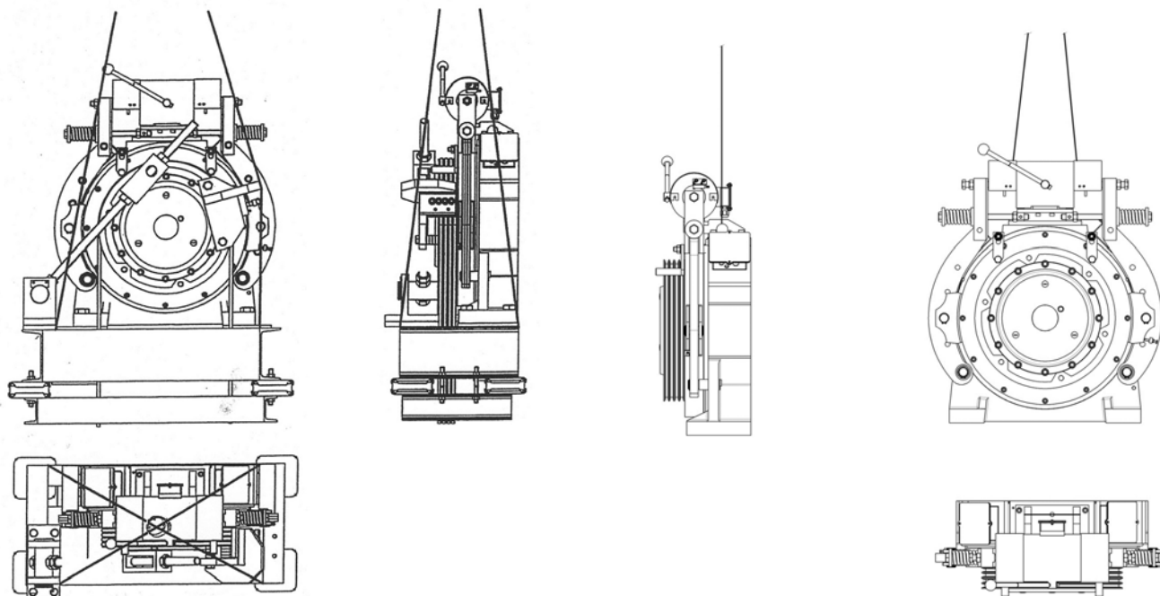
Рис. 18. Схема строповки
