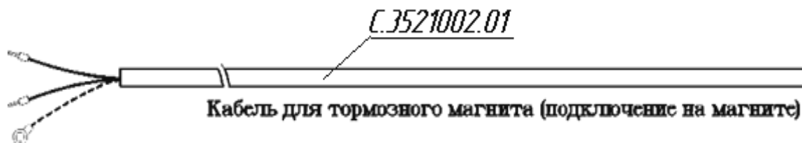
Рис. 11. Кабель питания электромагнита тормоза
