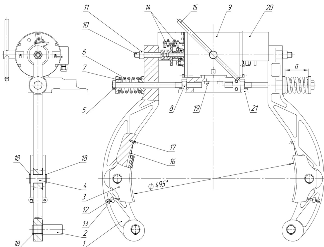
Рис. 24. Замена колодок
