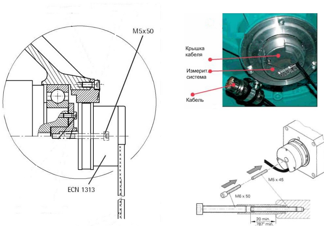
Рис. 27. Крепление энкодера.
